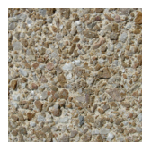
Calcaire jaune
